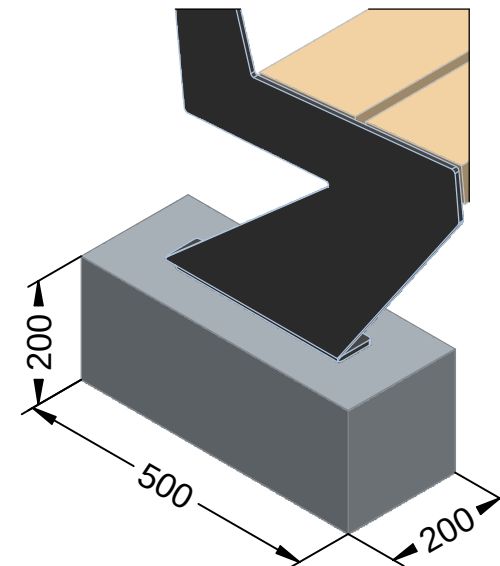
Detalle de anclaje
