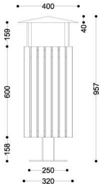
Rzut z boku/frontu
