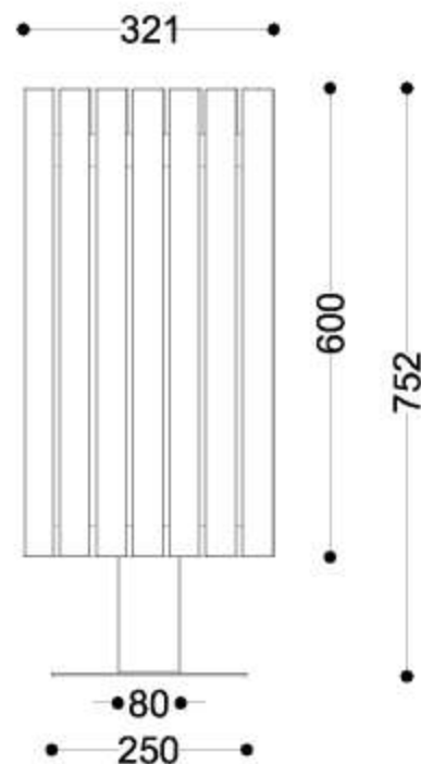
Rzut z boku
