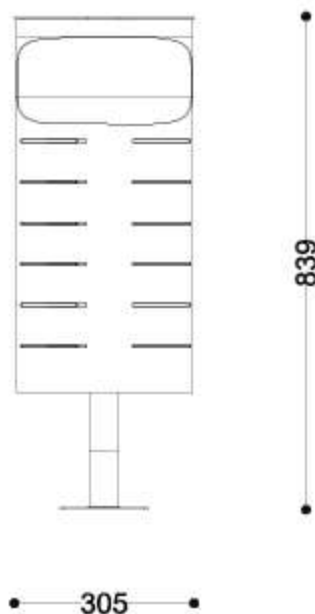
Rzut z frontu
