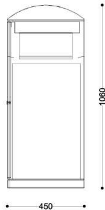
Rzut z boku
