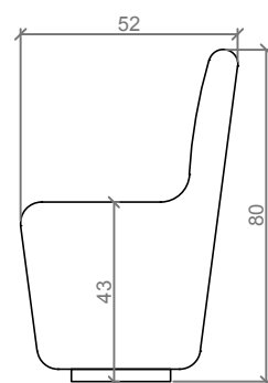
PERFIL / PROFILE
