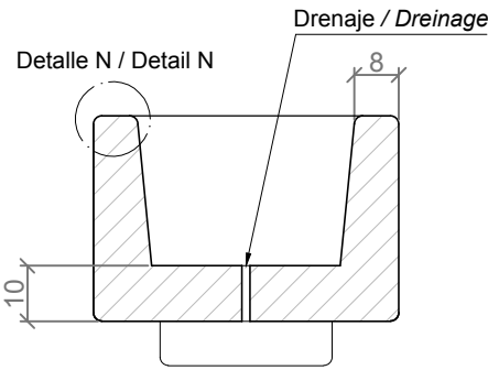
SECCIÓN A-A' / SECTION A-A'
