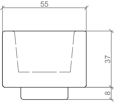
PERFIL / PROFILE
