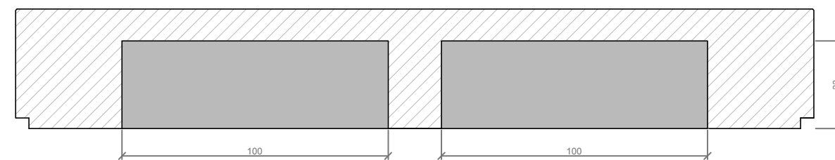
SECCIÓN A-A' / SECTION A-A'
