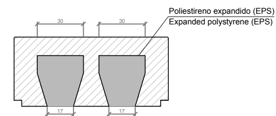
SECCIÓN B-B' / SECTION B-B'
