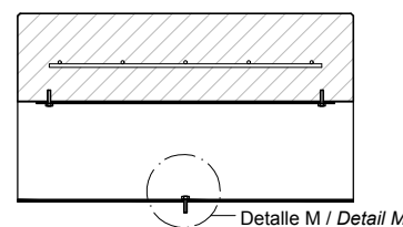
SECCIÓN B-B' / SECTION B-B'
