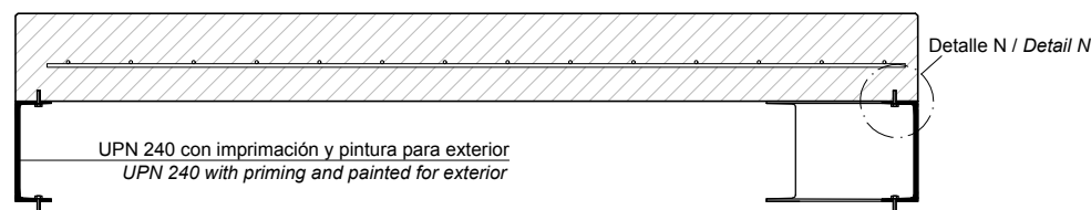
SECCIÓN A-A' / SECTION A-A'
