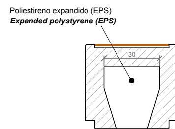
SECCIÓN B-B' / SECTION B-B'
