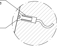
DETALLE M / DETAIL M Casquillo de elevación / Lifting sleeve
