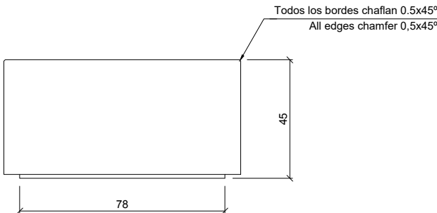
PERFIL / RIGHT SIDE
