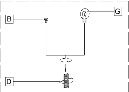
SISTEMA DE ELEVACIÓN / LIFTING SYSTEM
