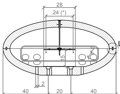
SECTION A-A' / SECTION A-A'
