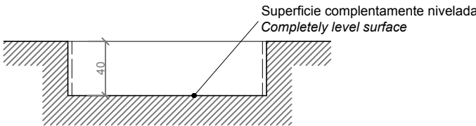
RASA EN SECCIÓN / SECTION
