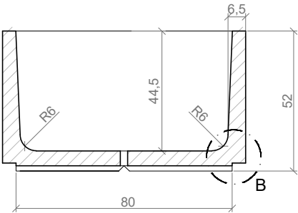
SECCIÓN A-A' / SECTION A-A'
