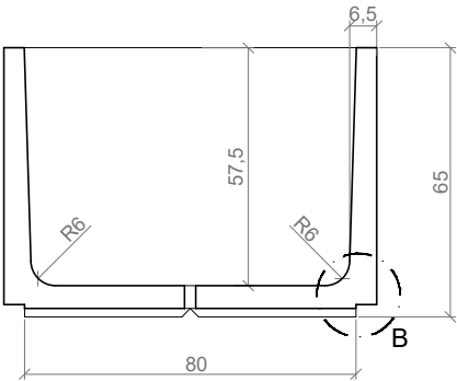
SECCIÓN A-A' / SECTION A-A'
