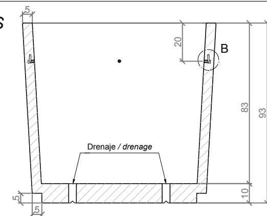
SECCIÓN A-A' / SECTION A-A'
