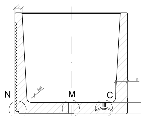
SECCIÓN A-A' / SECTION A-A'
