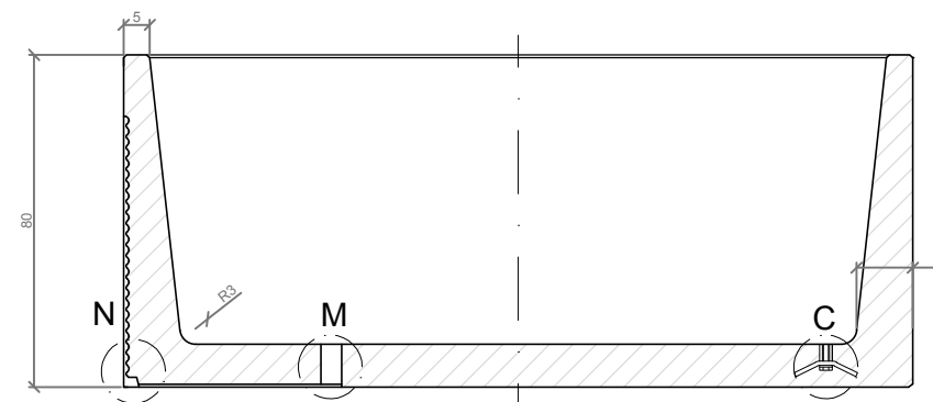
SECCIÓN A-A' / SECTION A-A'
