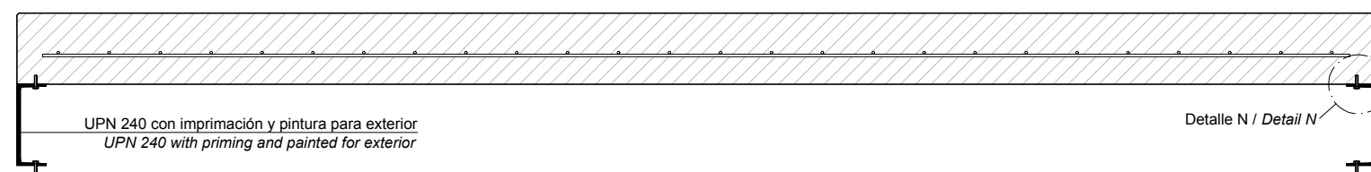
SECCIÓN A-A' / SECTION A-A'
