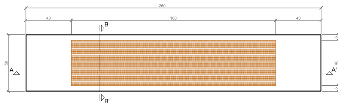
PLANTA / TOP VIEW
