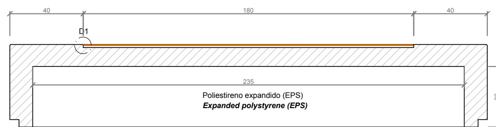
SECCIÓN A-A' / SECTION A-A'
