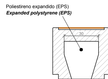
SECCIÓN B-B' / SECTION B-B'
