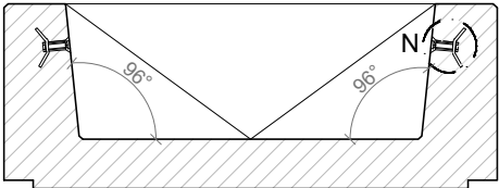
SECCIÓN A-A' / SECTION A-A'
