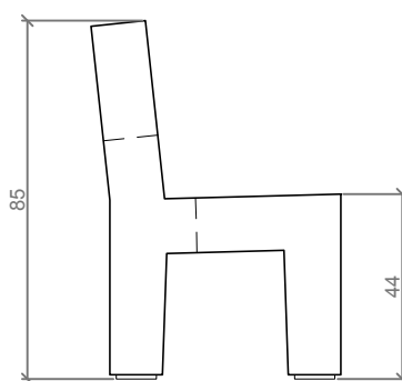
PERFIL / PROFILE
