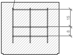
SECCIÓN B-B' / SECTION B-B'
