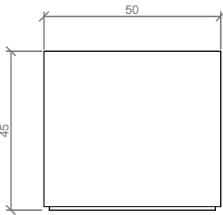
PERFIL / PROFIL VIEW
