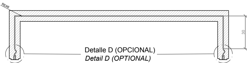
SECCIÓN A-A' / SECTION A-A'
