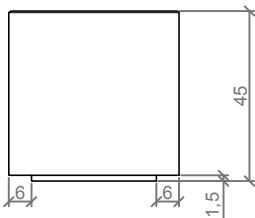
PERFIL / RIGHT SIDE
