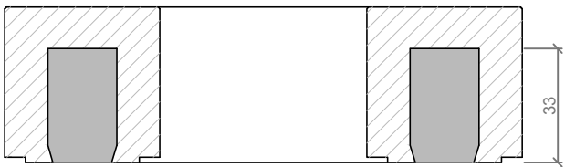
SECCIÓN A-A' / SECTION A-A'
