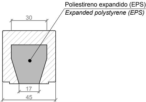
SECCIÓN B-B' / SECTION B-B'
