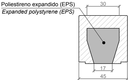
SECCIÓN B-B' / SECTION B-B'
