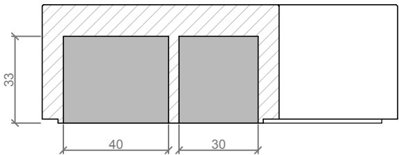
SECCIÓN A-A' / SECTION A-A'
