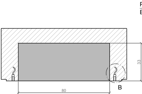
SECCIÓN A-A' / SECTION A-A'
