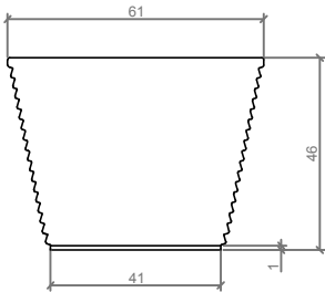
PERFIL / RIGHT SIDE
