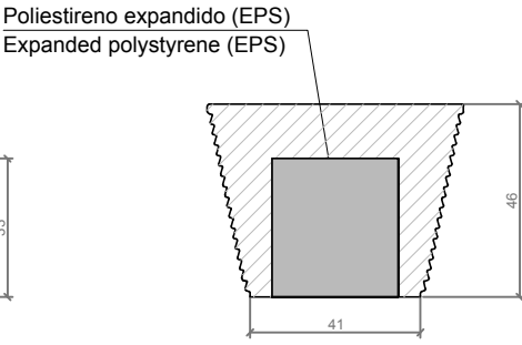
SECCIÓN B-B' / SECTION B-B'
