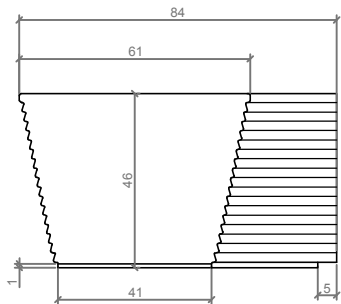
PERFIL / RIGHT SIDE
