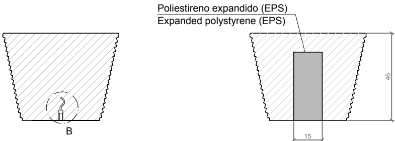
SECCIÓN A-A' / SECTION A-A'
