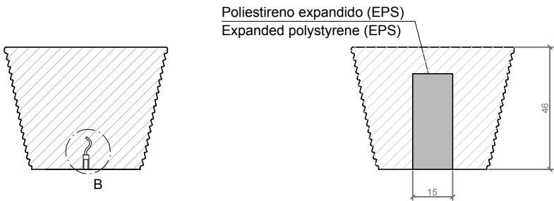
SECCIÓN A-A' / SECTION A-A'
