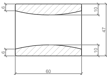
SECCIÓN A-A' / SECTION A-A'
