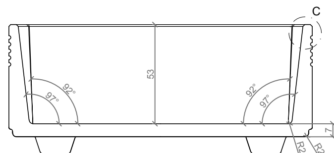
SECCIÓN A-A' / SECTION A-A'
