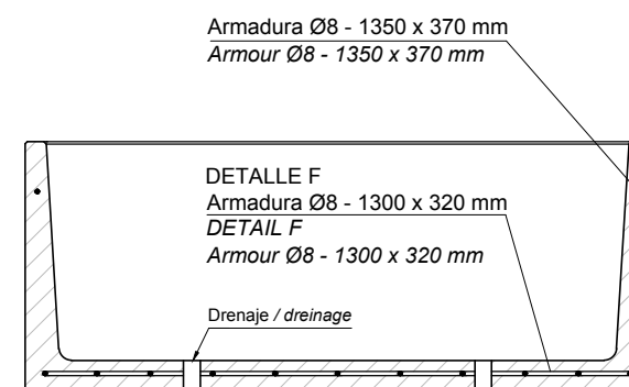
SECCIÓN B-B' / SECTION B-B'
