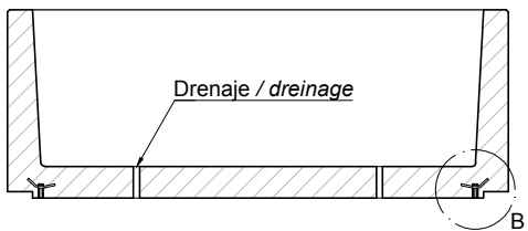
SECCIÓN A-A' / SECTION A-A'
