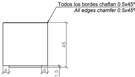
PERFIL / RIGHT SIDE
