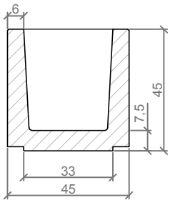
SECCIÓN B-B' / SECTION B-B'
