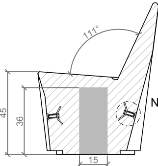
SECCIÓN B-B' / SECTION B-B'
