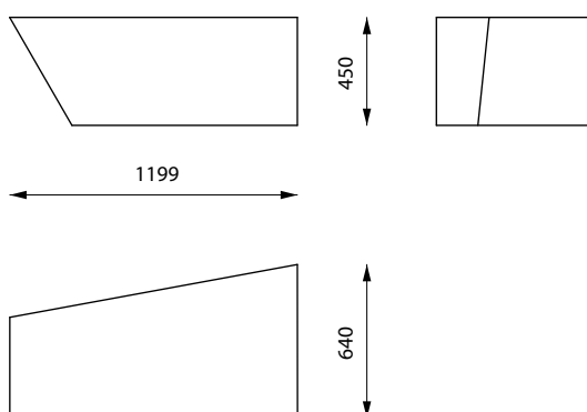
CRO-A2 330 kg
